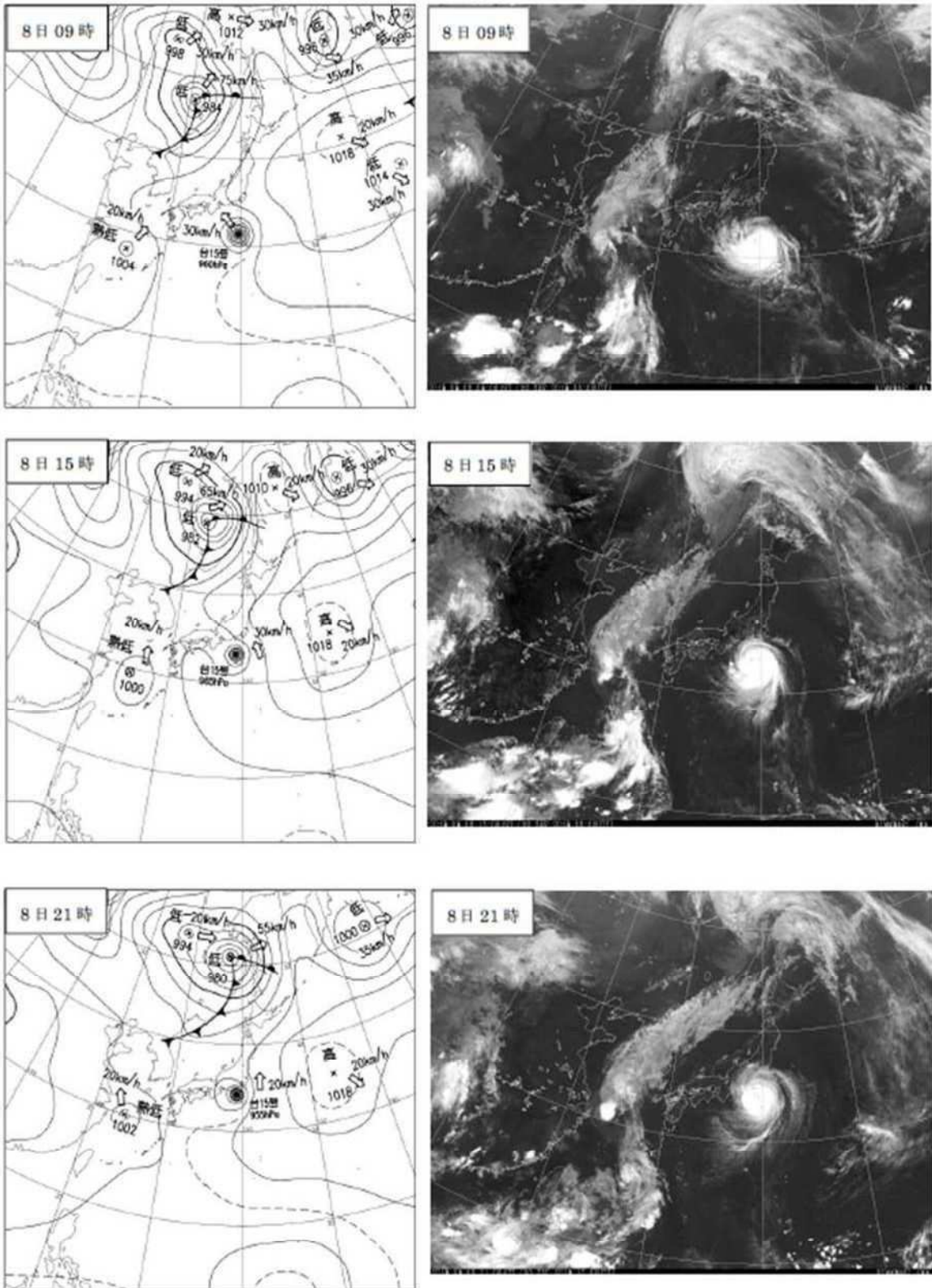
地上天気図・気象衛星赤外面像（令和元年9月8日09時～9日21時）
