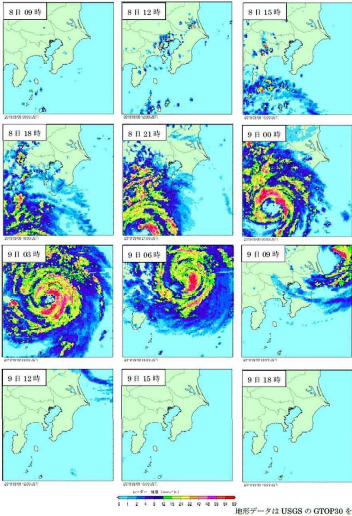
レーダーエコー合成図（令和元年 9 月 8 日 09 時～9 日 18 時）
