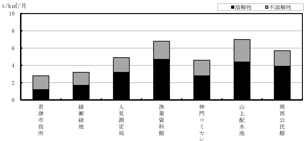
(図5-14) 降下ばいじん中の溶解性・不溶解性成分(年平均値)
