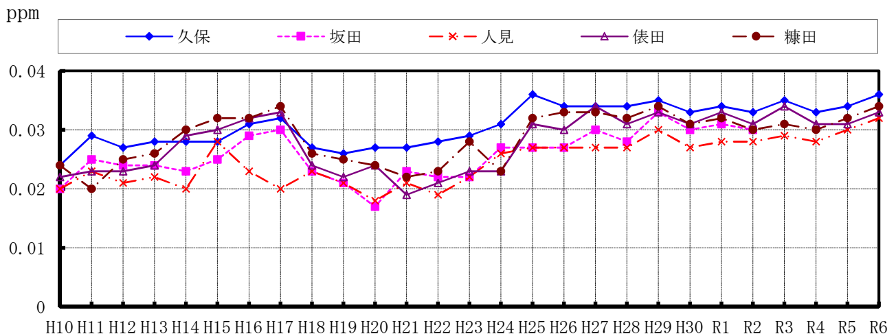
(図 5-6) 光化学オキシダント(昼間の1時間値の年平均値)の経年変化
