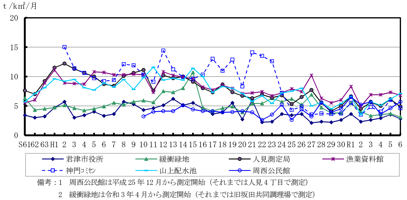
(図 5-15) 降下ばいじん量(年平均値)の経年変化
