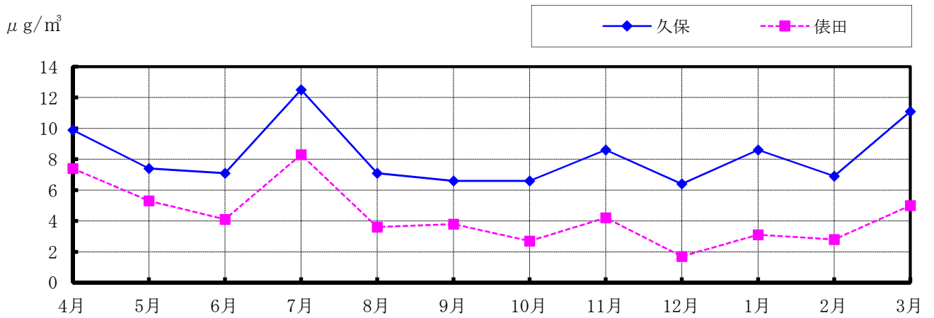
(図 5-18) 微小粒子状物質(月平均値)の月別推移
