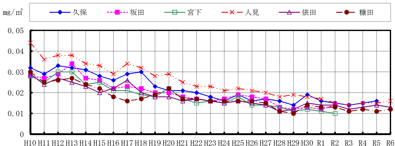
(図 5-8) 浮遊粒子状物質(年平均値)の経年変化
