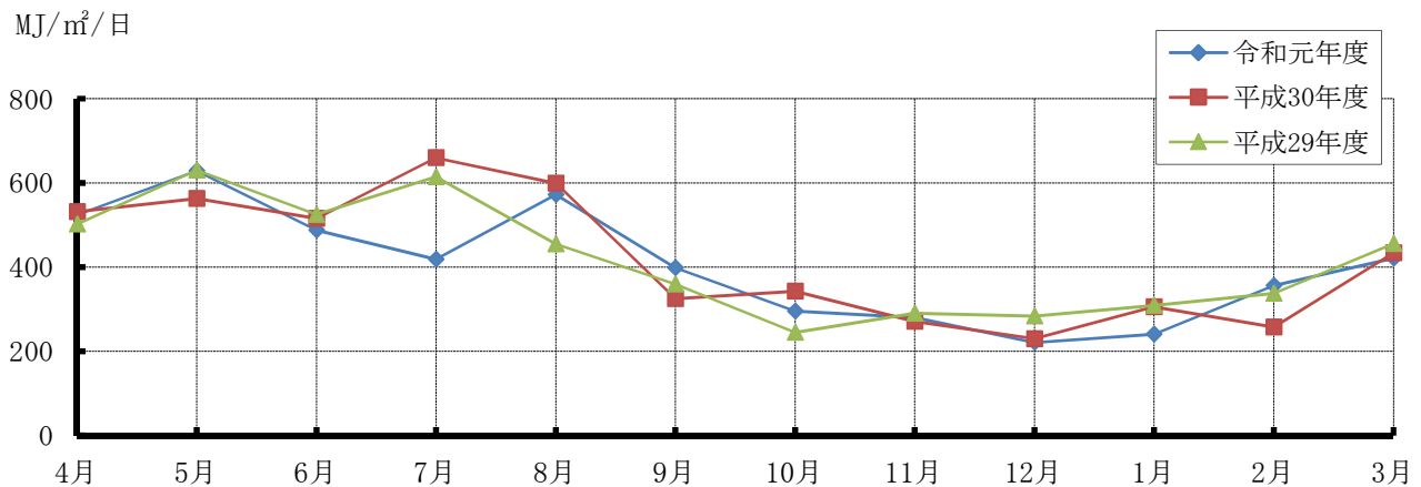
(図 4-4) 月間日射量の月別推移 (久保測定局)
