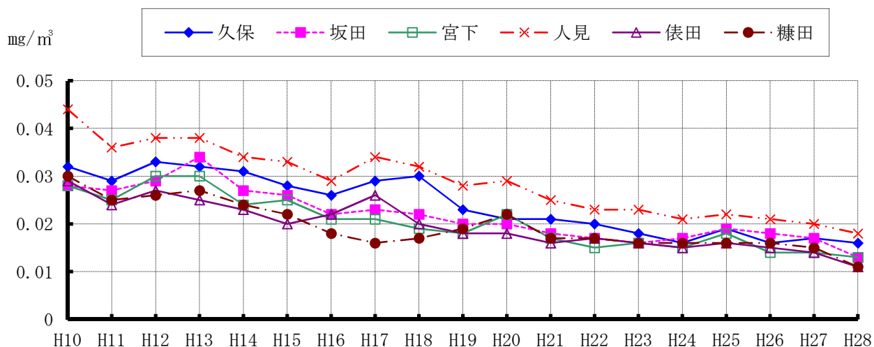
(図 5-8) 浮遊粒子状物質(年平均値)の経年変化
