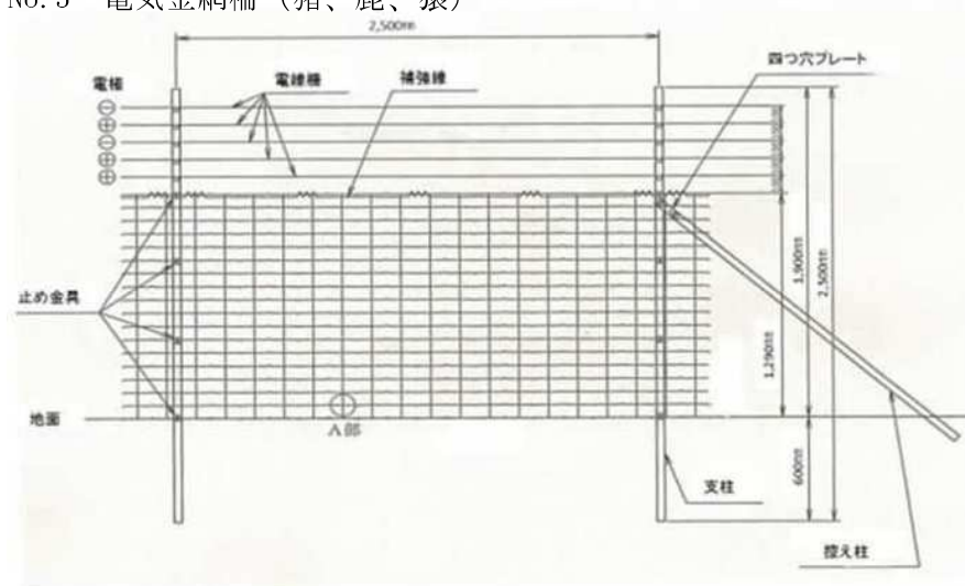
No. 5 電気金網柵 (猪、鹿、猿)
