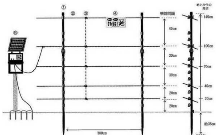
No. 2 電気柵（5段）
