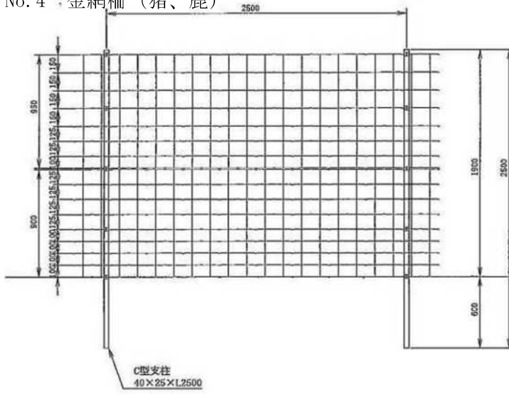
No. 4 金網柵 (猪、鹿)
