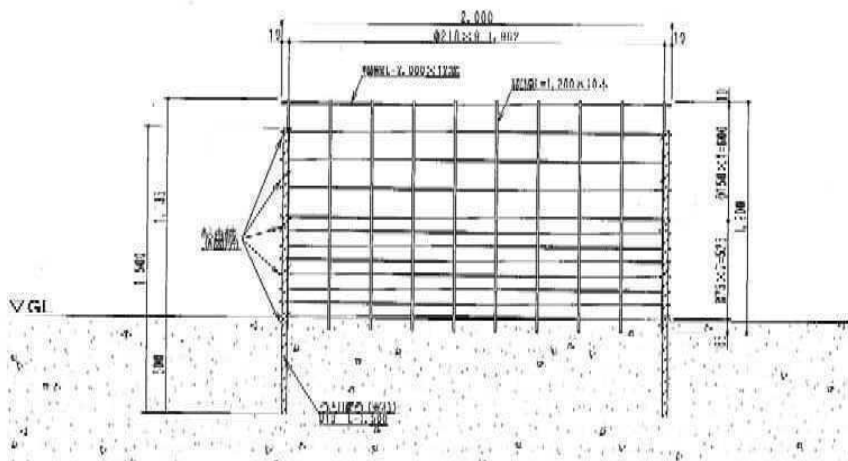
No. 6 ワイヤメッシュ (猪)
