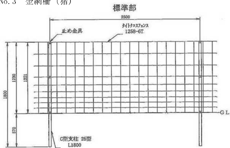
No. 3 金網柵（猪）
