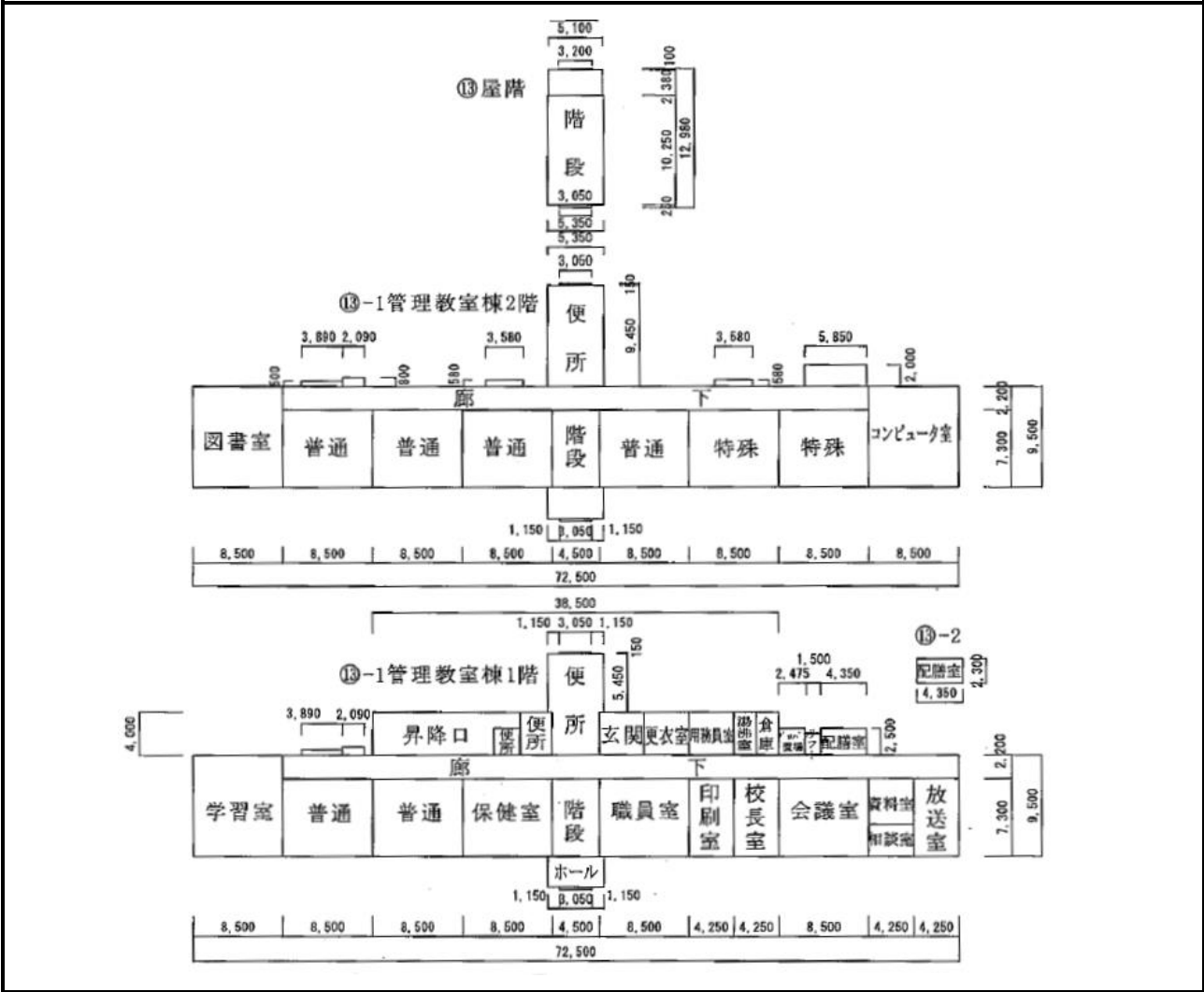
管理教室棟 平面図
