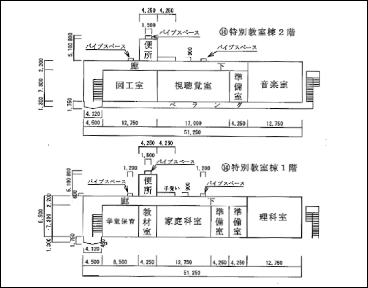
特別教室棟 平面図
