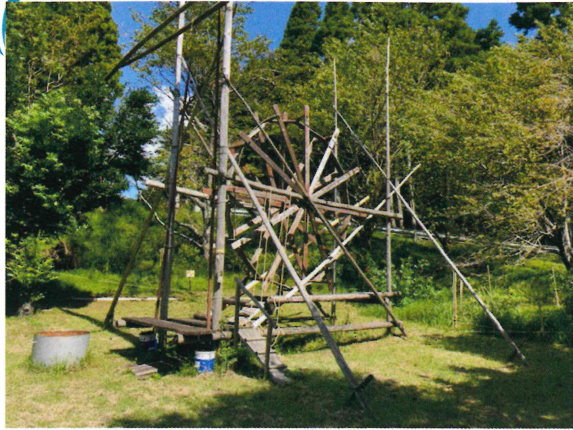
上総掘り井戸掘削の足場
