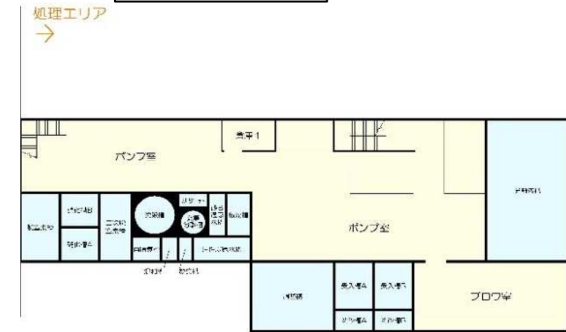
地下平面図
