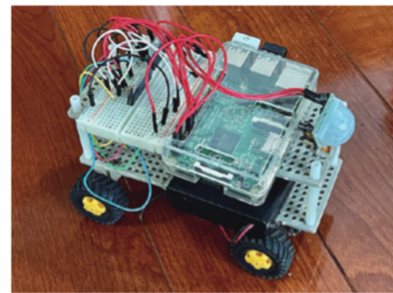
参考例：ハト対策ロボット ハトが来るとセンサーが反応して、ハトを追いかける
