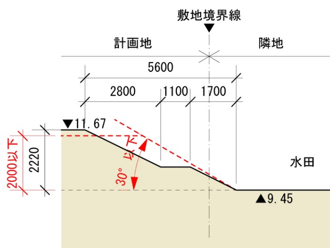
B-B' 法面現況断面イメージ
