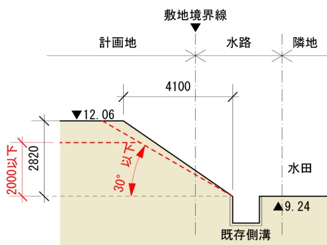
A-A' 法面現況断面イメージ
