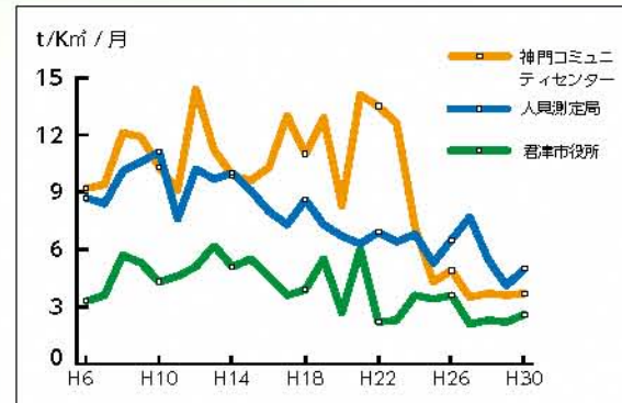
1カ月間で1Kmあたり何tの降下ばいじんが積もったかを示すグラフ
