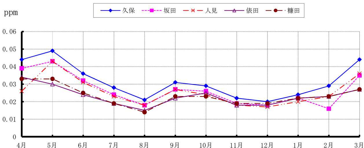
(図 5-17) 光化学オキシダントの月別推移(昼間の1時間値の月平均値)
