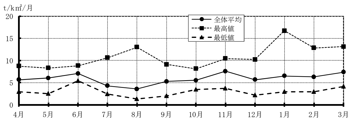
(図5-10) 全地点平均値による降下ばいじん量(総量)の月別推移
