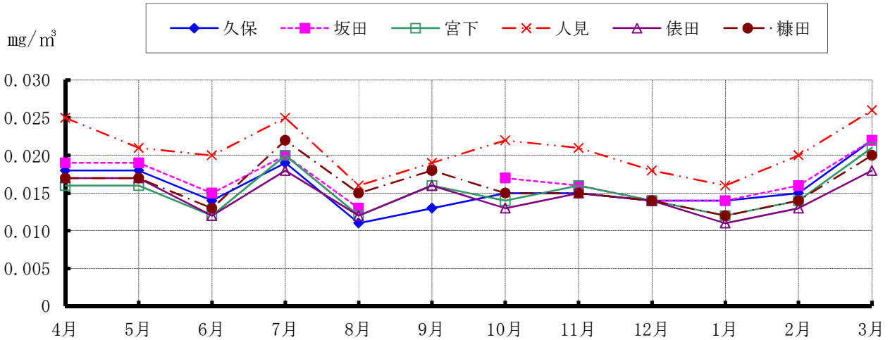
(図 5-5) 浮遊粒子状物質(月平均値)の月別推移
