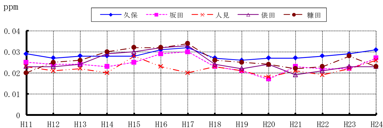
(図 5-16) 光化学オキシダント(昼間の 1 時間値の年平均値)の経年変化
