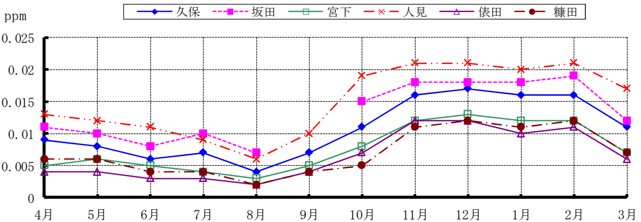
(図 5-15) 二酸化窒素(月平均値)の月別推移
