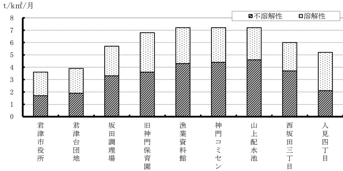
(図 5-12) 降下ばいじん量(年平均値)の経年変化
