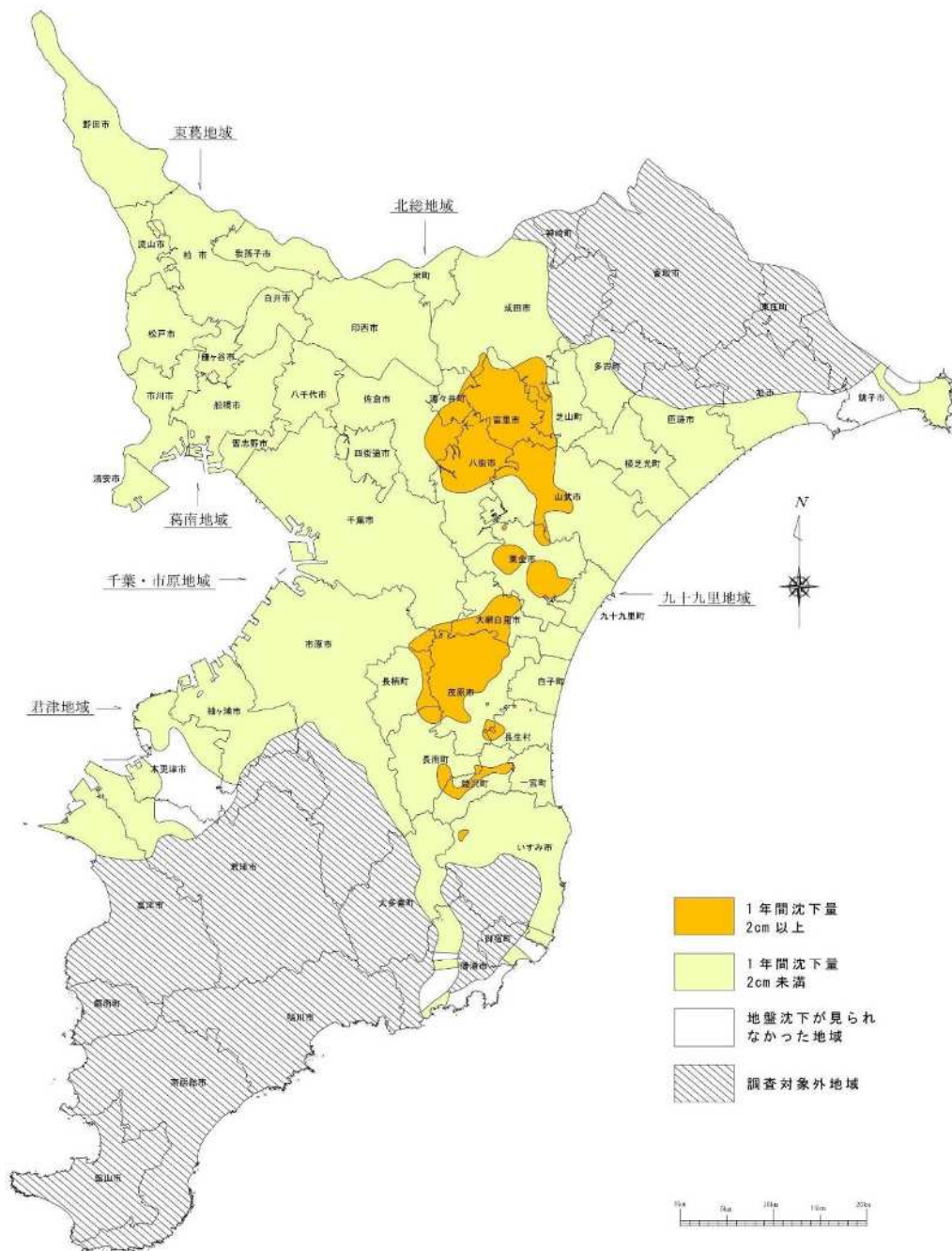
(図10-1) 千葉県水準基標変動図 (1年間変動図)
