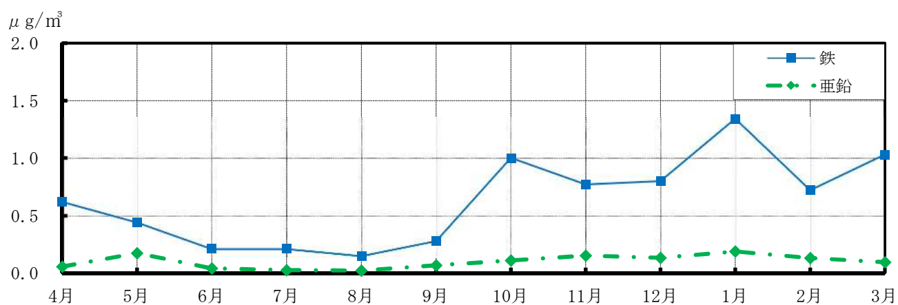
(図 5-11) 人見測定局における金属成分濃度の月別推移 鉄濃度・亜鉛濃度
