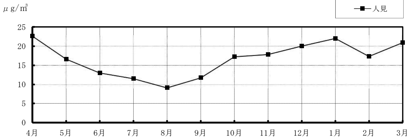
(図 5-10) 人見測定局における浮遊粒子状物質濃度 (SPM) の月別推移
