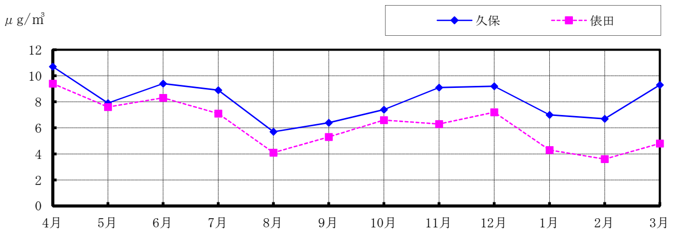
(図 5-18) 微小粒子状物質(月平均値)の月別推移
