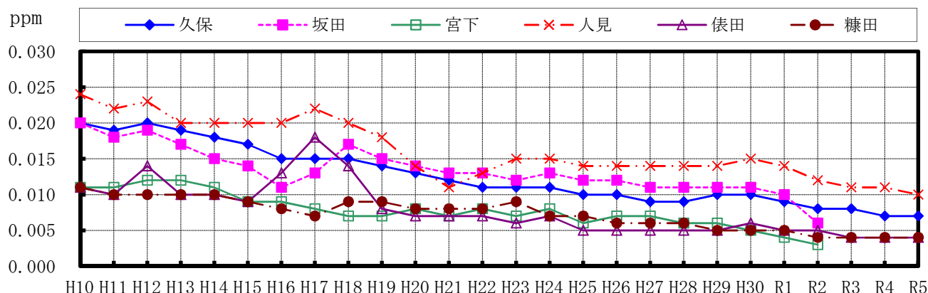
(図 5-4) 二酸化窒素(年平均値)の経年変化
