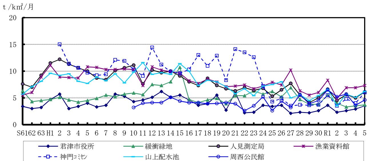
(図 5-15) 降下ばいじん量(年平均値)の経年変化
