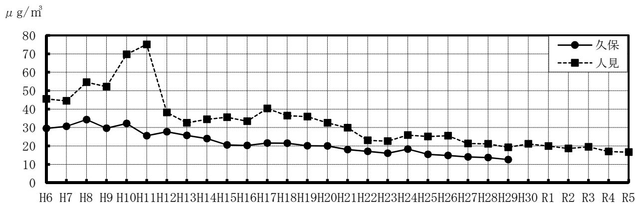
(図 5-13) 浮遊粒子状物質濃度(年平均値)の経年変化
