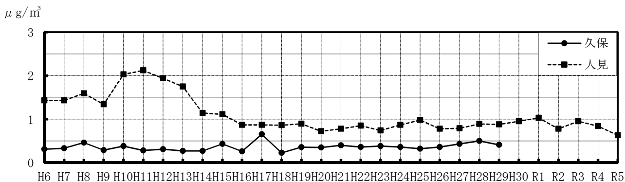
(図 5-12) 主な金属成分濃度(年平均値)の経年変化
