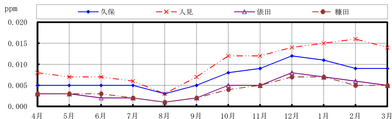
(図 5-5) 二酸化窒素(月平均値)の月別推移
