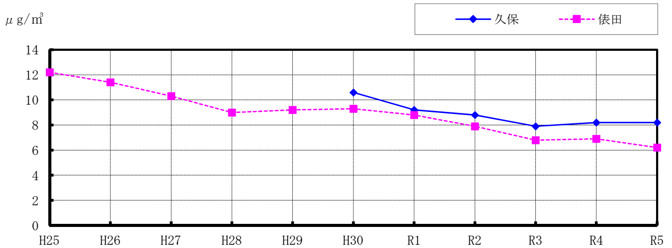
(図 5-17) 微小粒子状物質(年平均値)の経年変化
