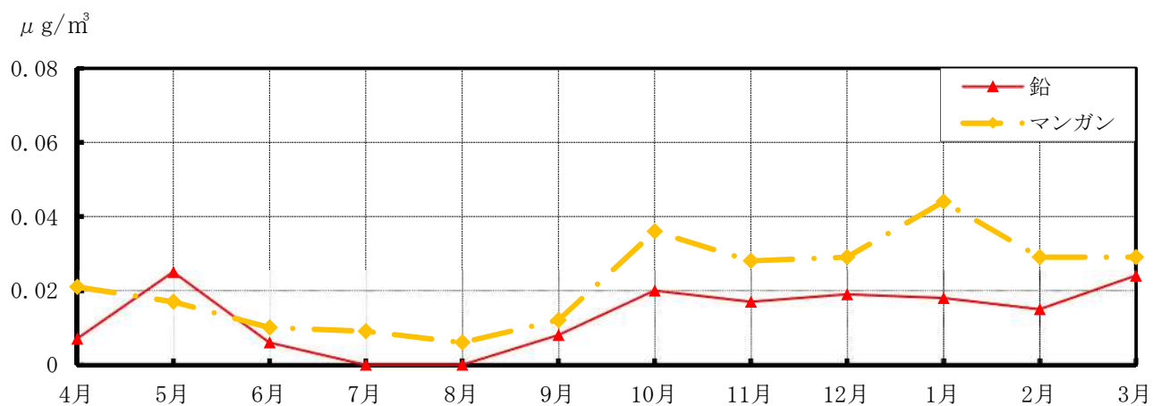
鉛濃度・マンガン濃度
