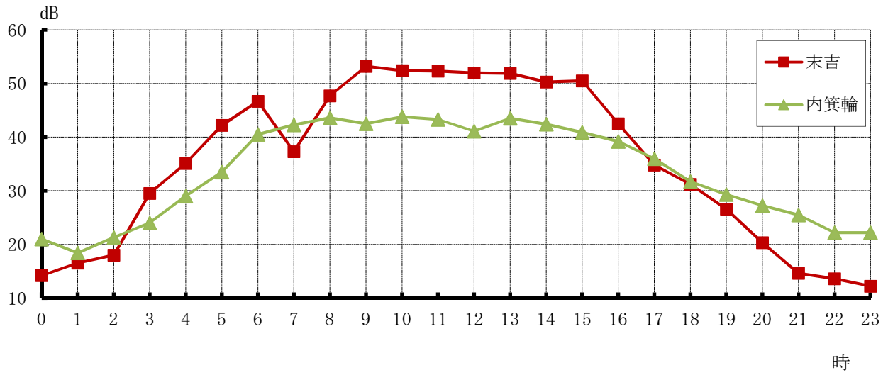
(圖 11-5) 道路交通振動經時變化
