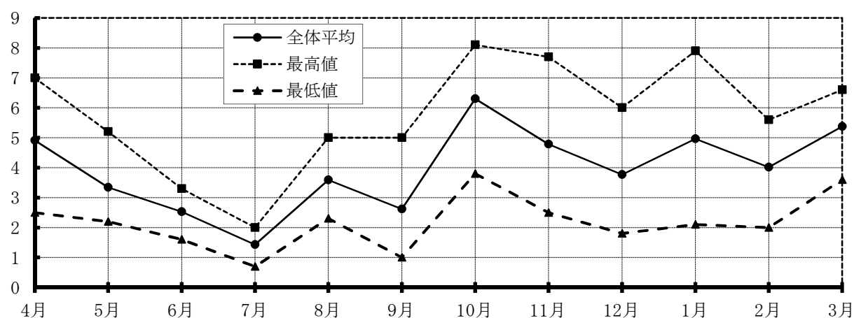
(図 5-14) 全地点の平均値による降下ばいじん量(総量)の月別推移
