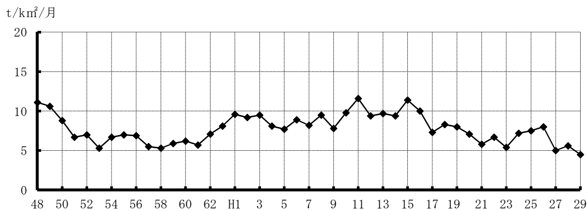
(図 5-17) 山上配水池における降下ばいじん量の経年変化
